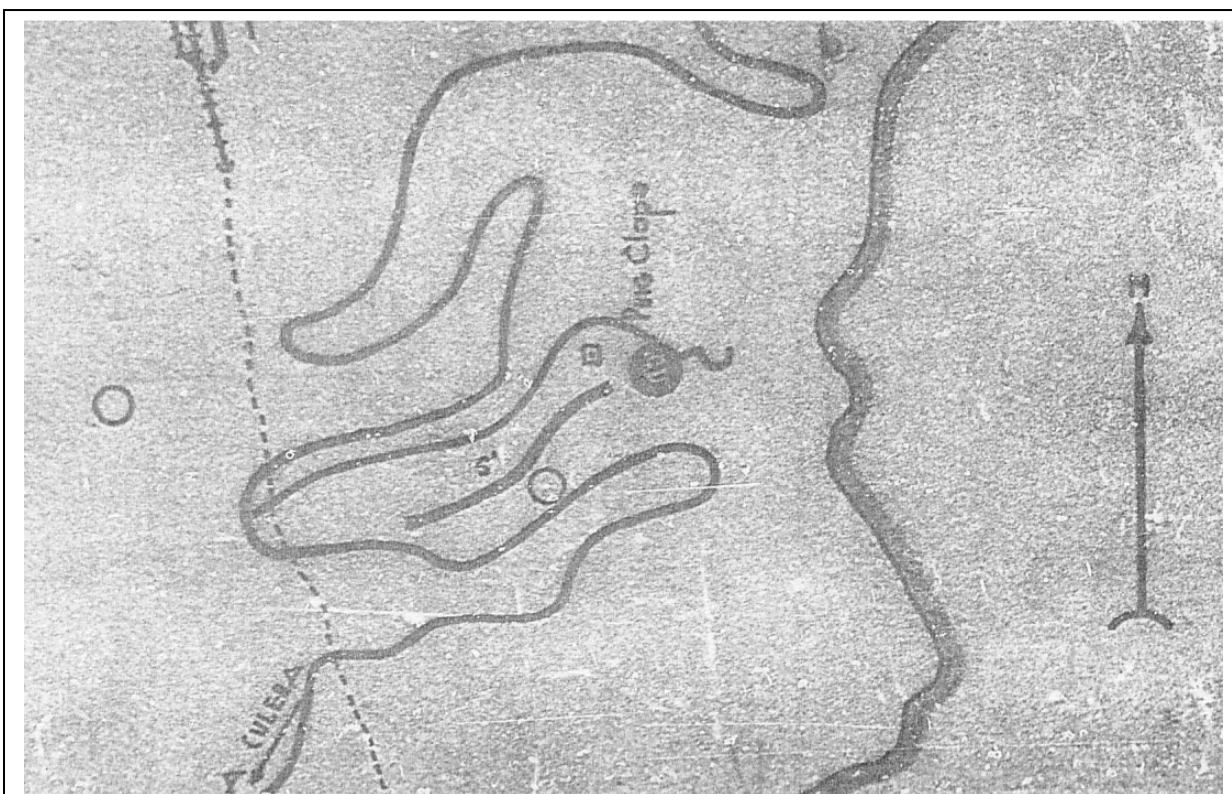
Detalle de un plano de la Agrupación Norte de Defensa de Costas que muestra la situación de la batería de Puig Clapé. Se aprecia la pista construida, todavía existente desde la carretera hasta el asentamiento de los cañones. También se puede ver una obra de defensa y el polvorín de la batería a ras de la carretera en la vertiente de Colera. La construcción de una antena de telecomunicaciones destruyó los pozos al lado de la batería de Puig Clapé, no hace muchos años.
